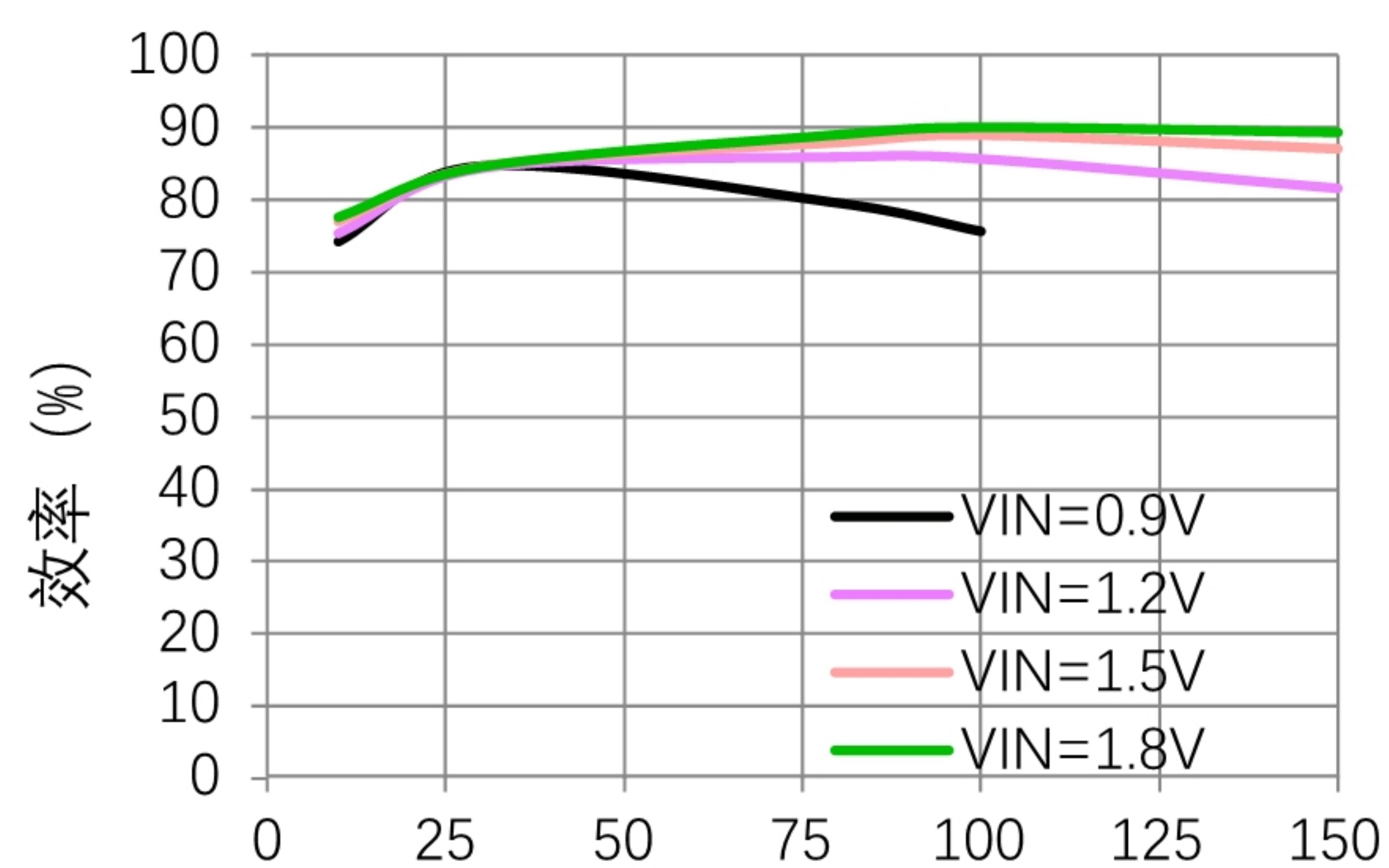
输出电流与效率关系
