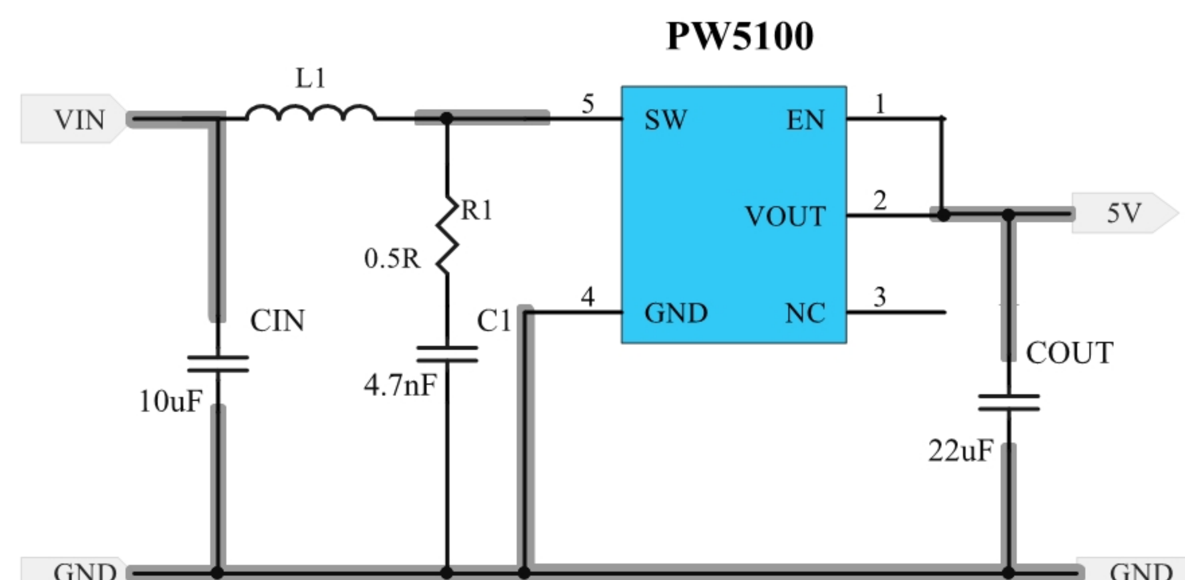
图 2：典型应用电路图：5V（增加RC电路）
