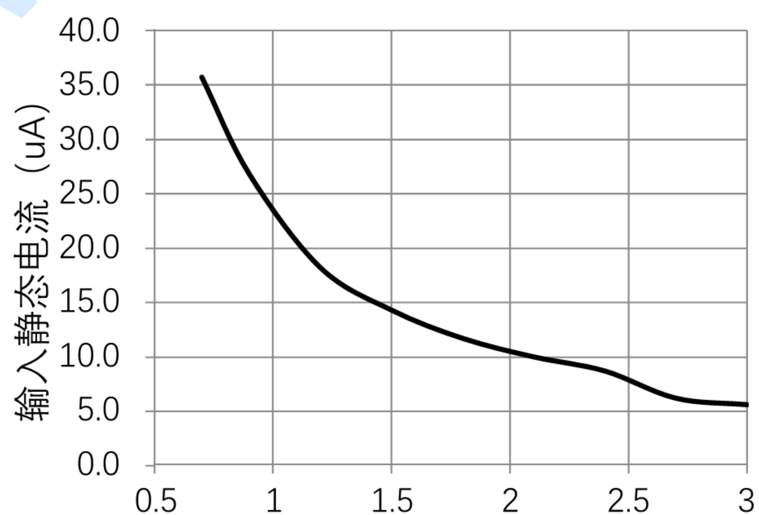
静态电流与输入电压关系
