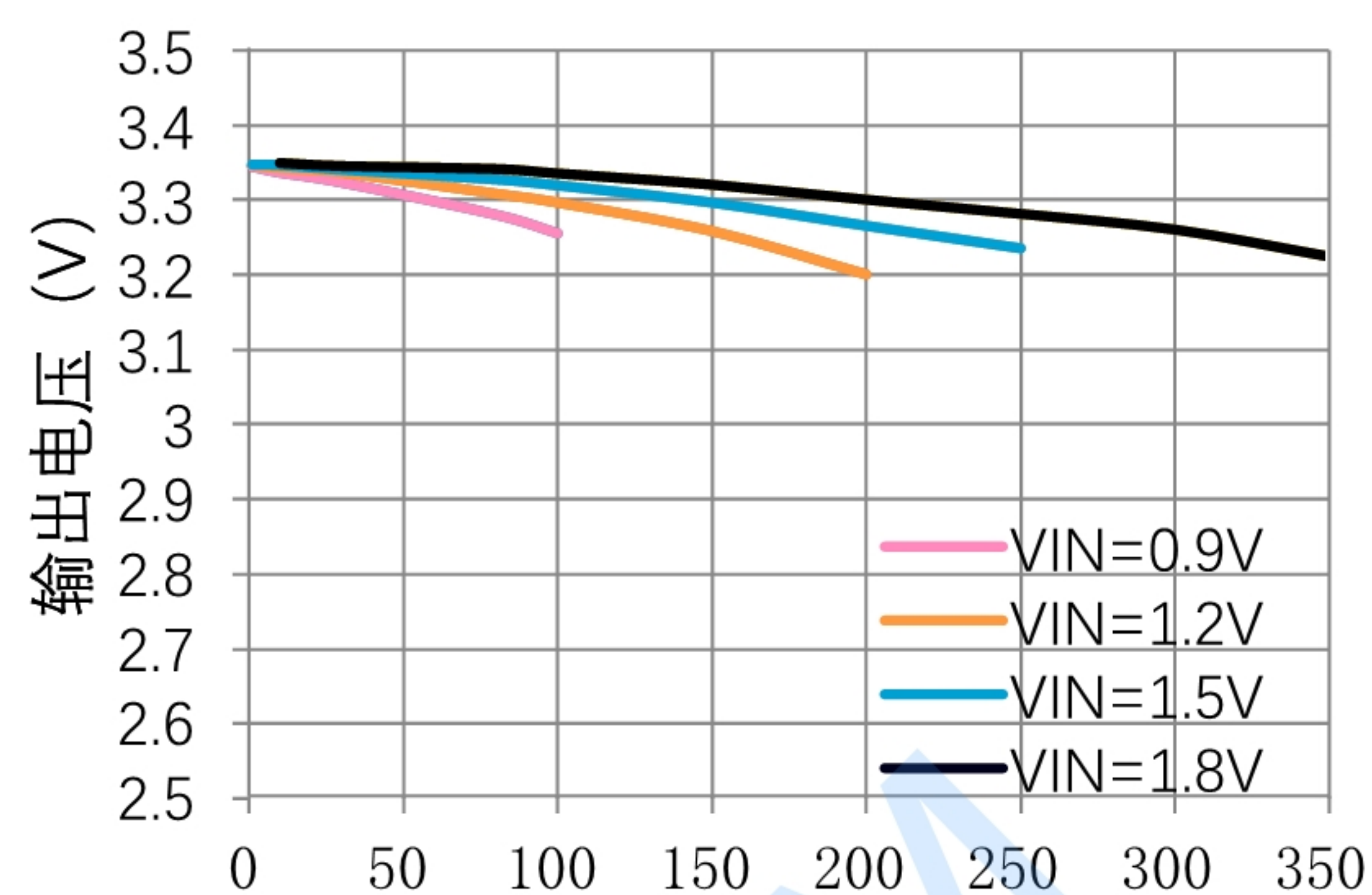
输出电压与输出电流
